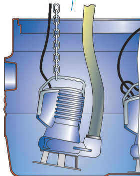
Preparación para el vaciado de emergencia mediante una llave de paso o una bomba auxiliar
