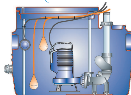
Posibilidad de instalación para bombas de alimentación horizontal mediante un pie de acoplamiento fijado en el fondo. La estanqueidad está garantizada por un elemento especial con O-ring.
